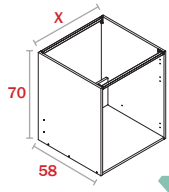
Módulo Fregadero B70
