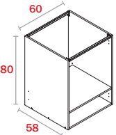
Módulo Inferior Horno B80
