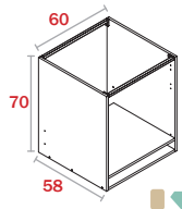
Módulo Horno B70
