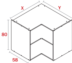
Módulo Esquina "L" B80
