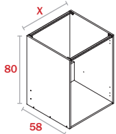
Módulo Inferior Fregadero B80
