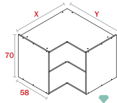
Módulo Esquina "L" B70
