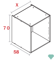
Módulo Cajonero B70
